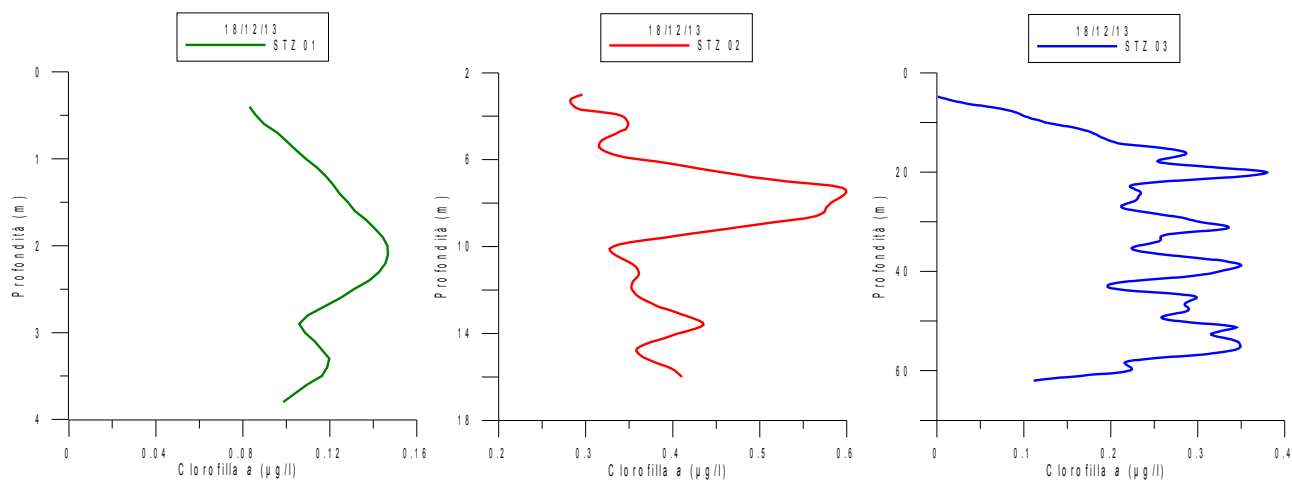
Fig. 9 Andamento della Clorofilla a nelle Stazioni ST01PT, ST02PT, ST03PT durante le campagne FPOA_4
