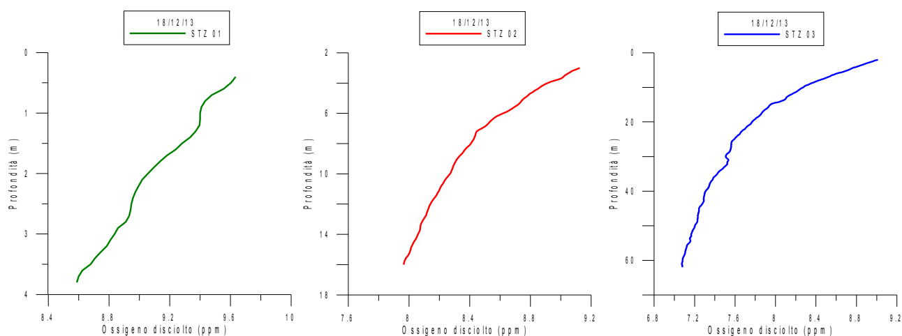
Fig. 8 Andamento dell'Ossigeno disciolto nelle Stazioni ST01PT, ST02PT, ST03PT durante le campagne FPOA_4
