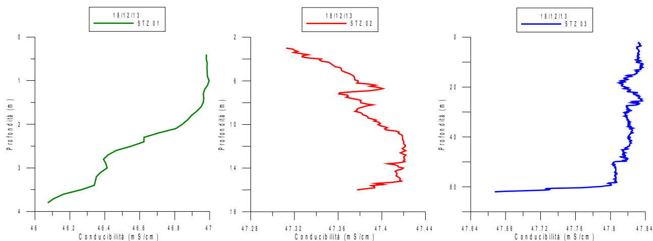
Fig. 5 Andamento della Conducibilità nelle Stazioni ST01PT, ST02PT, ST03PT durante le campagne FPOA_4
