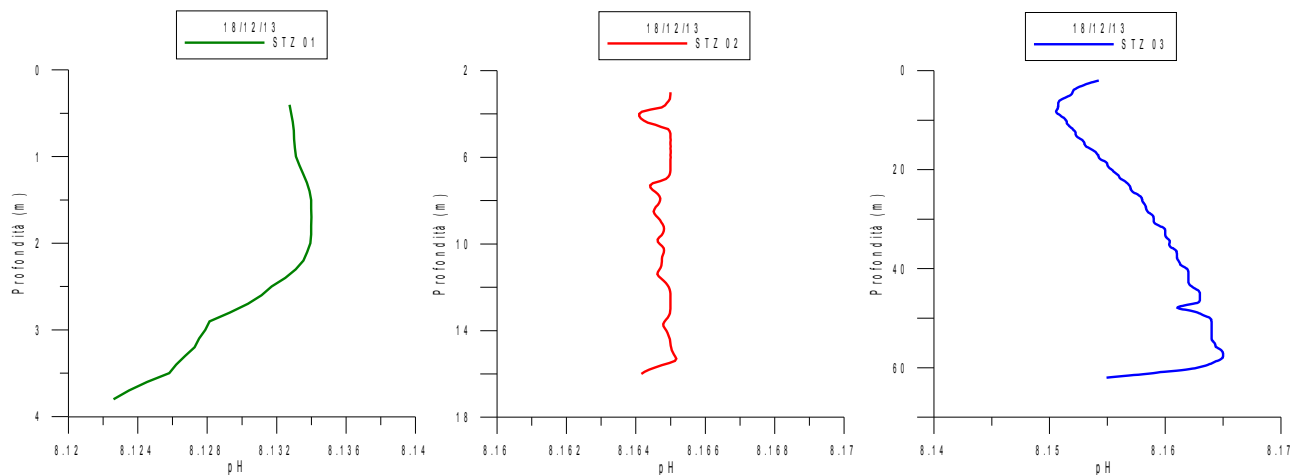
Fig. 7 Andamento della pH nelle Stazioni ST01PT, ST02PT, ST03PT durante le campagne FPOA_4
