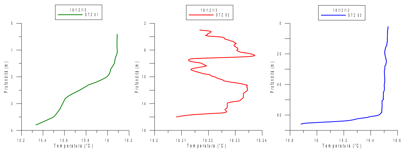
Fig. 4 Andamento della Temperatura nelle Stazioni ST01PT, ST02PT, ST03PT durante le campagne FPOA_4
